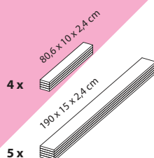
Bauteil SF-L (lange Seitenfläche)
